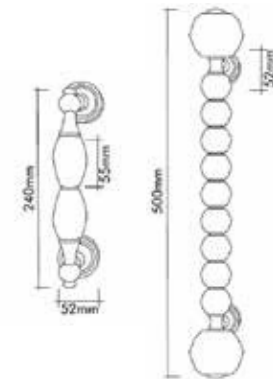
10437-520-2 Chrome / Krom
